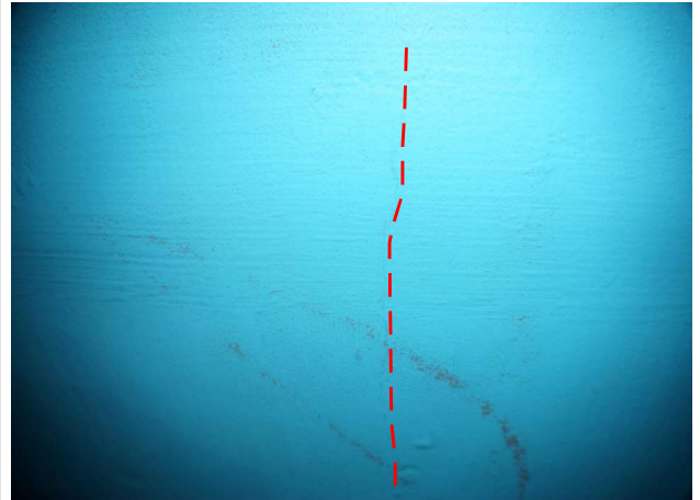
배수지1지 벽체 균열(0.3mm미만)
