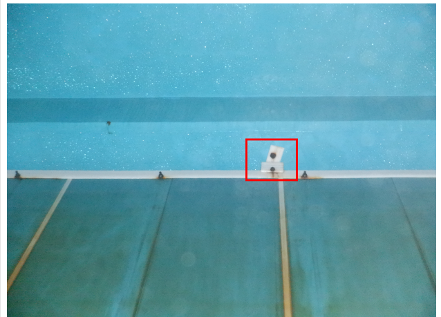
배수지1지 기둥 녹, 부식
