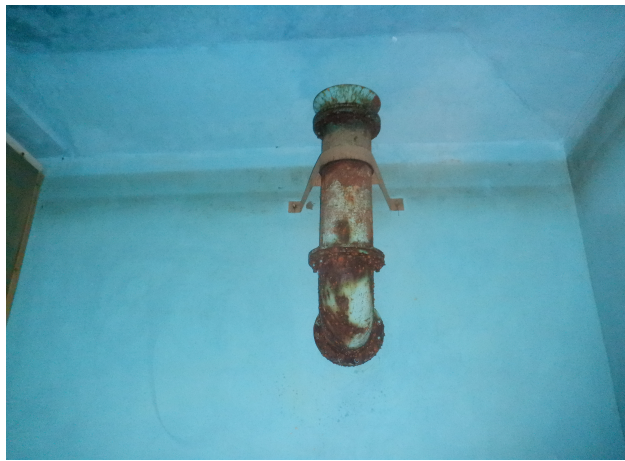
2지 유입배관 관부식
